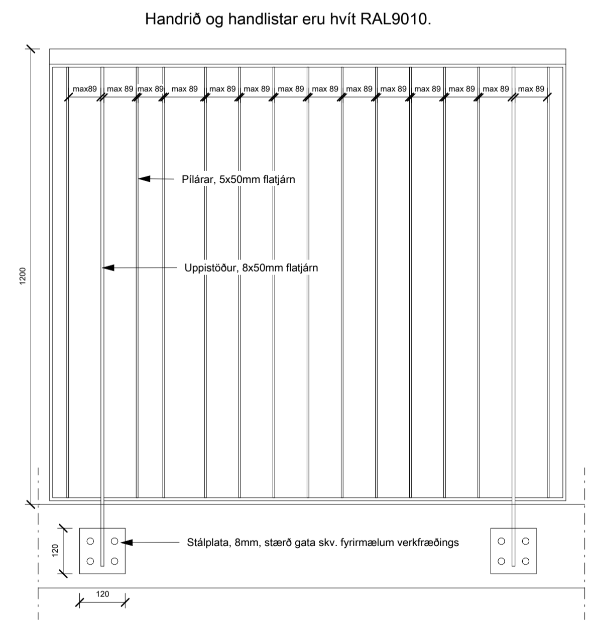
HANDRÍÐ - PRINSIPP ÚTLIT HANDRÍÐA VIÐ OP EFSTU HÆÐAR mkv: 1 : 10
