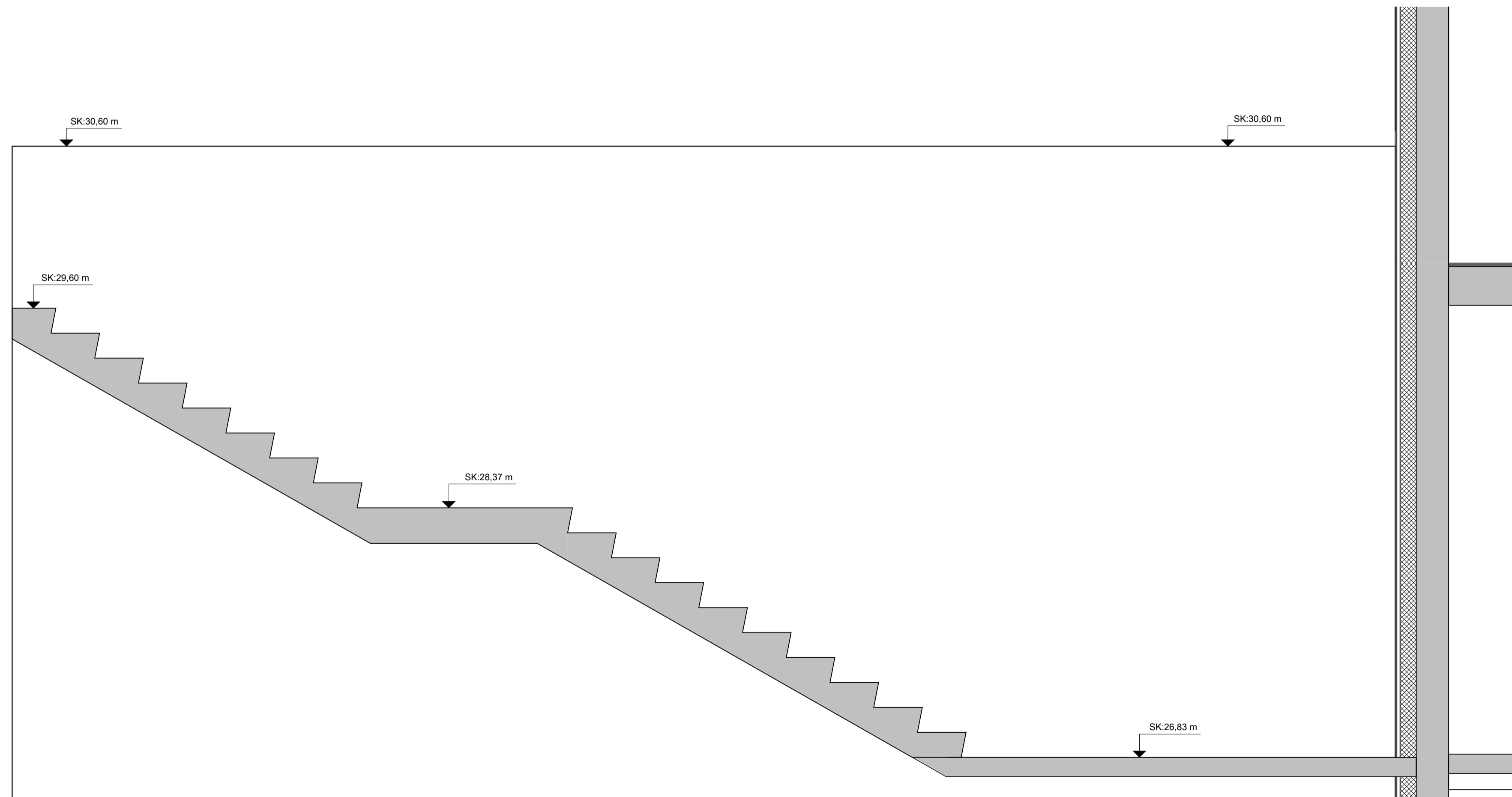
Snið B-B flóttastigi mkv: 1 : 20
