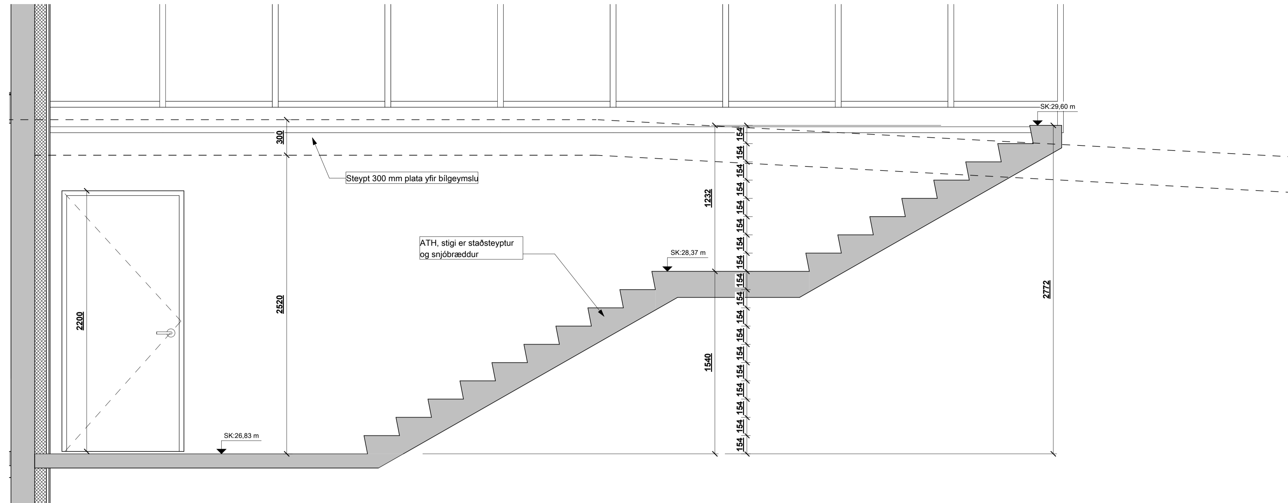
Snið A-A flóttastigi mkv: 1 : 20
