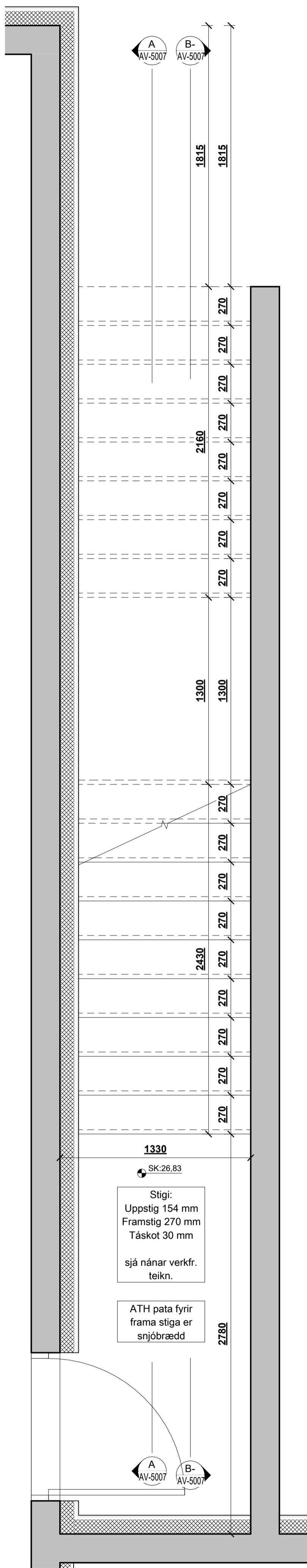
Grunnmynd - flóttastigi mkv: 1 : 20
